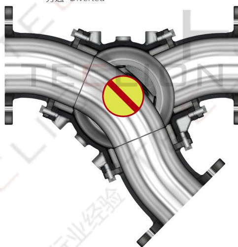
旁通 Diverted
